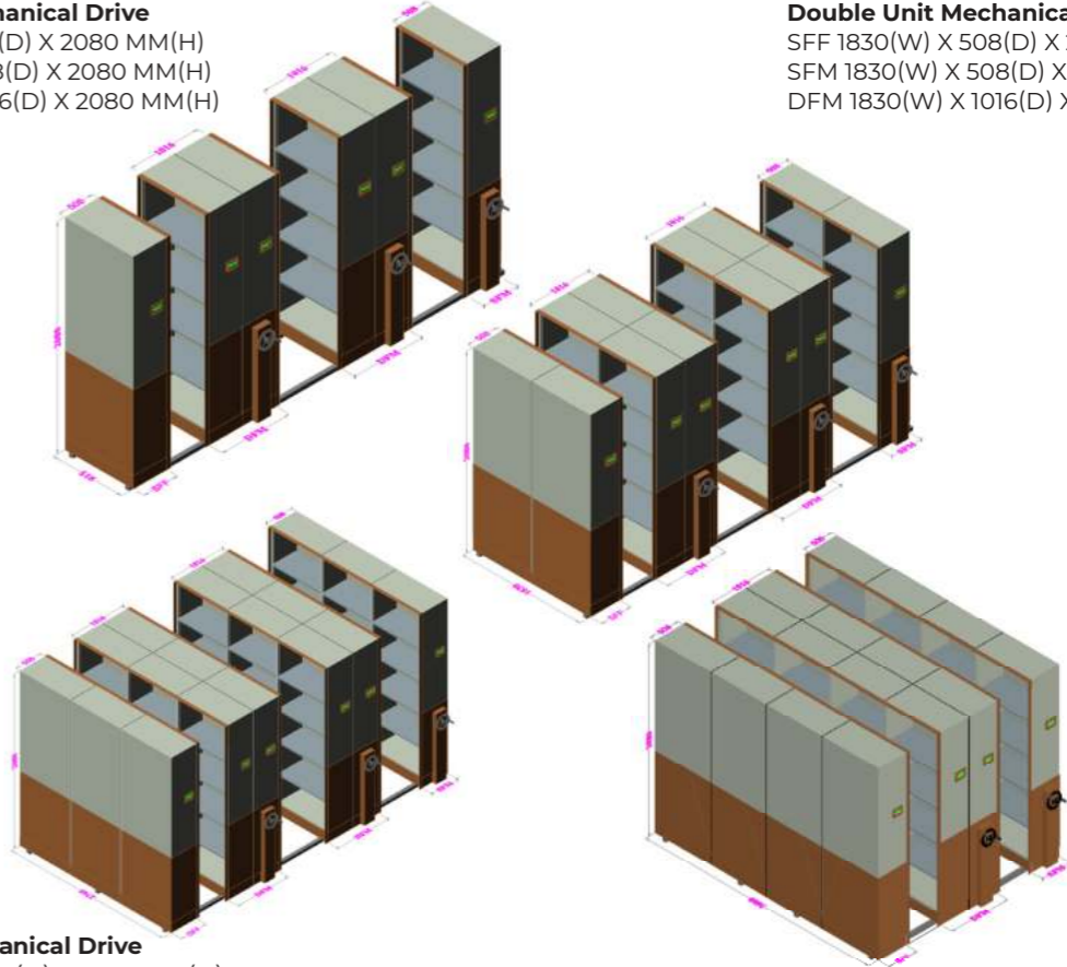
Quad Unit Mechanical Drive SFF 3660(W) X 508(D) X 2080 MM(H) SFM 3660(W) X 508(D) X 2080 MM(H) DFM 3660(W) X 1016(D) X 2080 MM(H)
